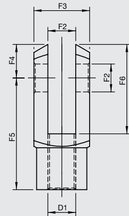
RC ROD CLEVIS
