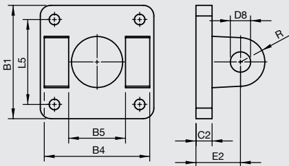
SF SWIVEL FLANGE
