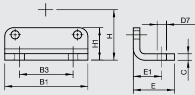
SF SWIVEL FLANGE
